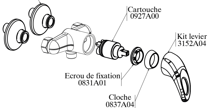
Ensemble rosace+excentrique 0898A00
